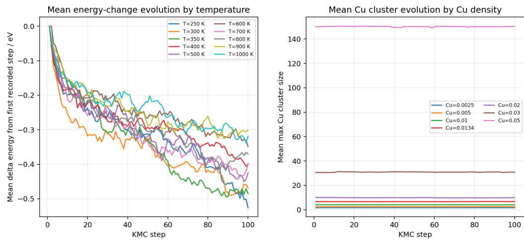
图 1: 材料能量变化与 Cu 团簇演化曲线
